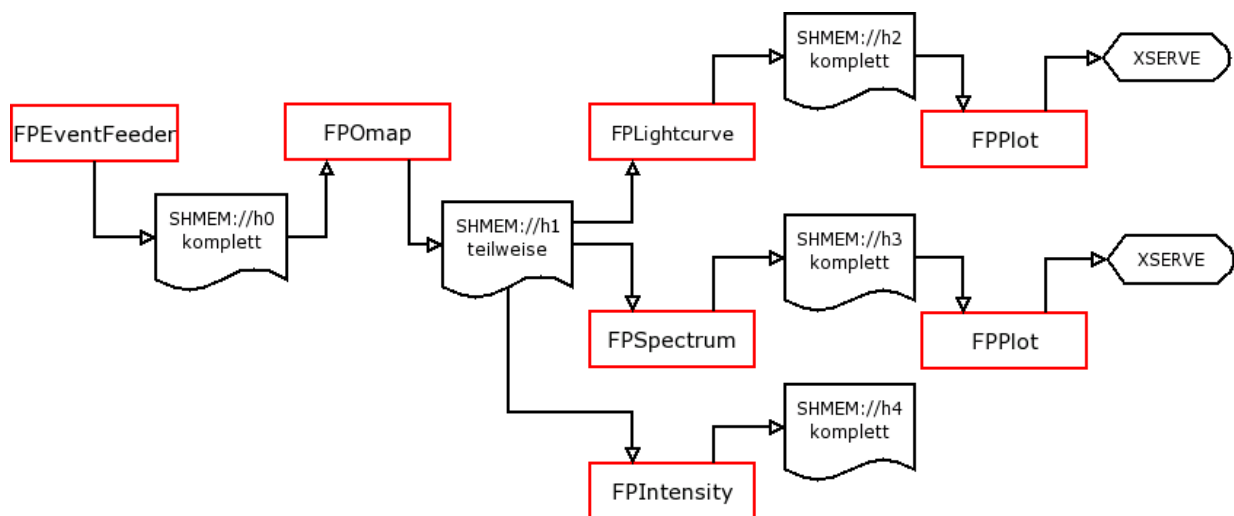
Abbildung 4.1: Die hier dargestellte Pipeline ist als Datei in meiner Software enthalten.
