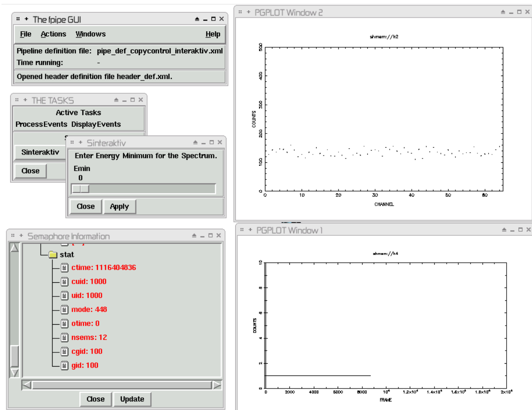
Abbildung 4.6: Screenshot des Programms mit interaktiver Pipelinedefinition
